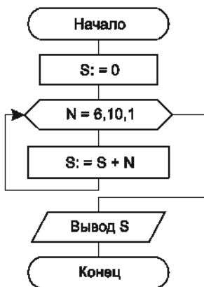
Рис. 6.3. Блок-схема алгоритма вычисления суммы чисел от 6 до 10
