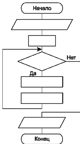
Рис. 7.6. «Слепая» блок-схема алгоритма вычисления произведения двух чисел с использованием только операции сложения
