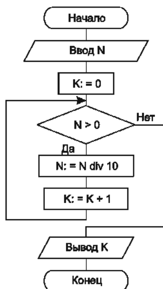
Рис. 7.12. Блок-схема алгоритма подсчета количества десятичных разрядов в заданном положительном числе N
