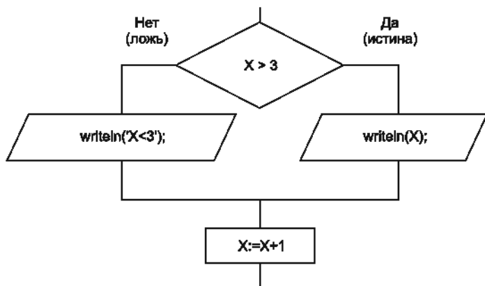
Рис. 5.2. Блок-схема алгоритма, выводящего число, если оно больше трех, или сообщение « X < 3 » в противном случае
