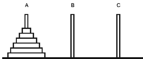
Рис. 20.2. Ханойские башни
