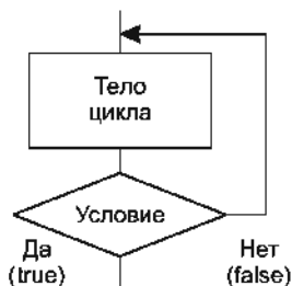
Рис. 7.8. Блок-схема цикла с постусловием
